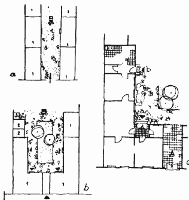
Сл. 12 — Комплекси станова у дворишту: а) два тракта станова покрај суседа (1); б) станови с лица и бочно поред суседа (2 шупа, 3 клозет); в) велики стан са крилом
