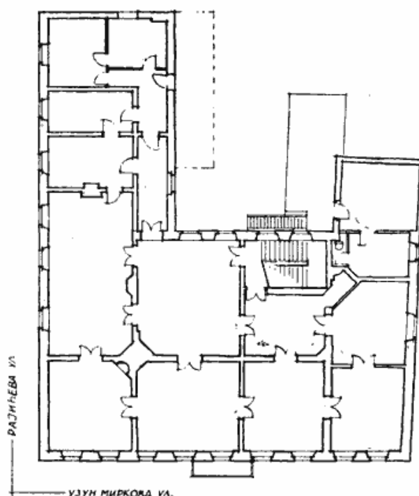
Сл. 5 — Оријенталски тип основе: лево, основа Ичкове куће (по Б. Којићу); десно, кућа Томе Вучића-Перишића (снимак Градског музеја)
