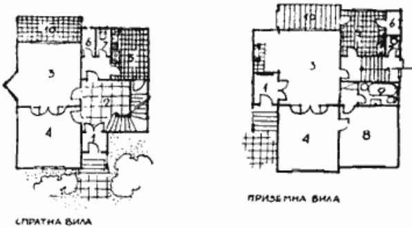
Сл. 26 — Мале виле. 1 улаз, 2 хол, 3 трпезарија, 4 комбинована соба, 5 кујна, 6 оства, 7 W. C., 8 спаваћа соба, 9 купатило, 10 тераса
