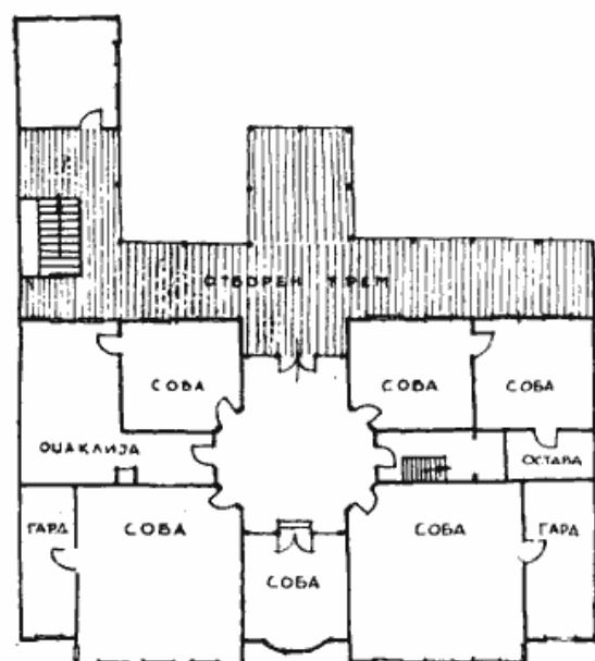
Сл. 5 — Оријенталски тип основе: лево, основа Ичкове куће (по Б. Којићу); десно, кућа Томе Вучића-Перишића (снимак Градског музеја)
