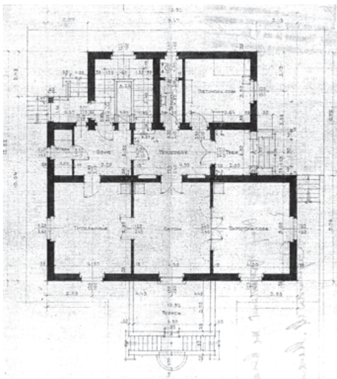
Сл. 4 / Инж. Цвејко Анђелковић, неизведени пројекат виле Даринке Михаиловић у Љубици Бојдана 22, основа приземља, 1939. (извор: ИАБ, ОГБ, ТД, ф–XXI–22–1939)
