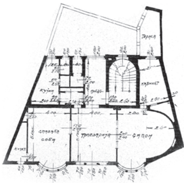
Сл. 1 / Арх. Бранислав Којић, пројекат породичне куће у Задарској 6, основа сјаја, 1926. (извор: ИАБ, ОГБ, ТД, ф-ХVI-55-1926)
