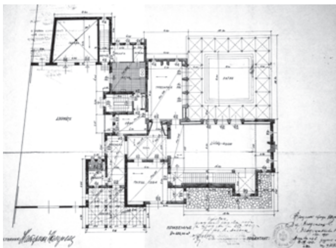
Сл. 6 / Арх. Владислав Владисављевић, пројекат виле Касидолац, основа пројекта, 1937. (извор: ИАБ, ОГБ, ТД, ф-XXIX-18-1937)
