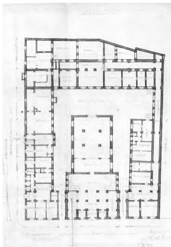
Слика 2. Женска учитељска школа, скица приземља
