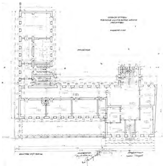
Слика 8. Женска учитељска школа, основа приземља
