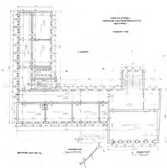
Слика 10. Женска учитељска школа, основа другог спрата
