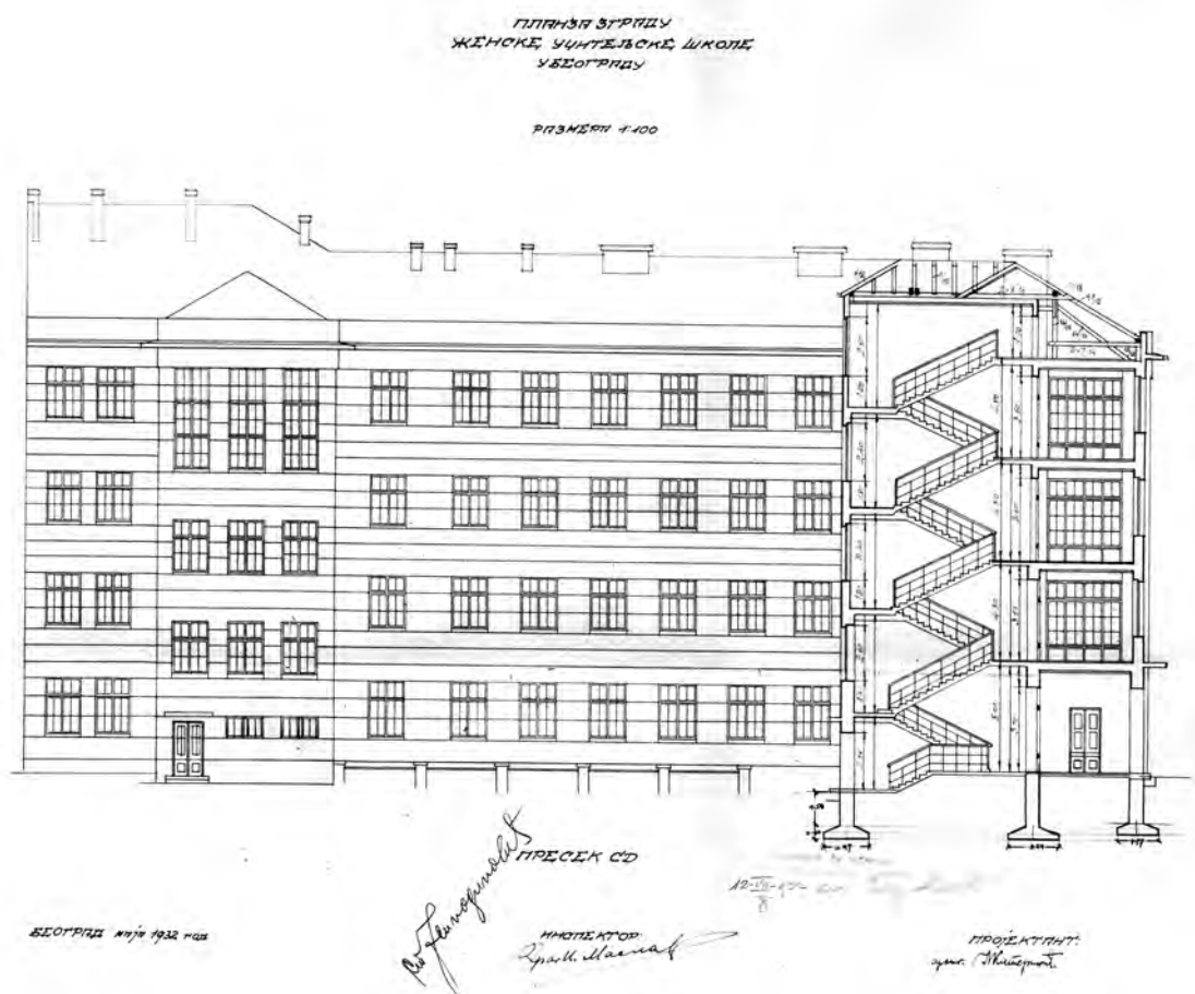
Слика 15. Интернат Женске учитељске школе, пресек Fig. 15 Boarding section of the Pegagogical School for Girls, section view
