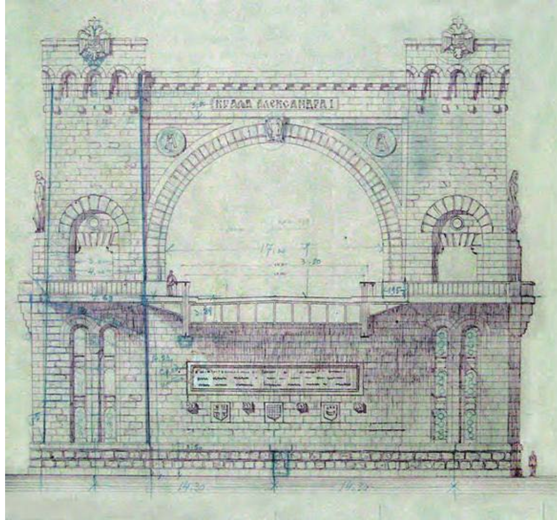
Николај Краснов, пилони моста краља Александра, 1930.
