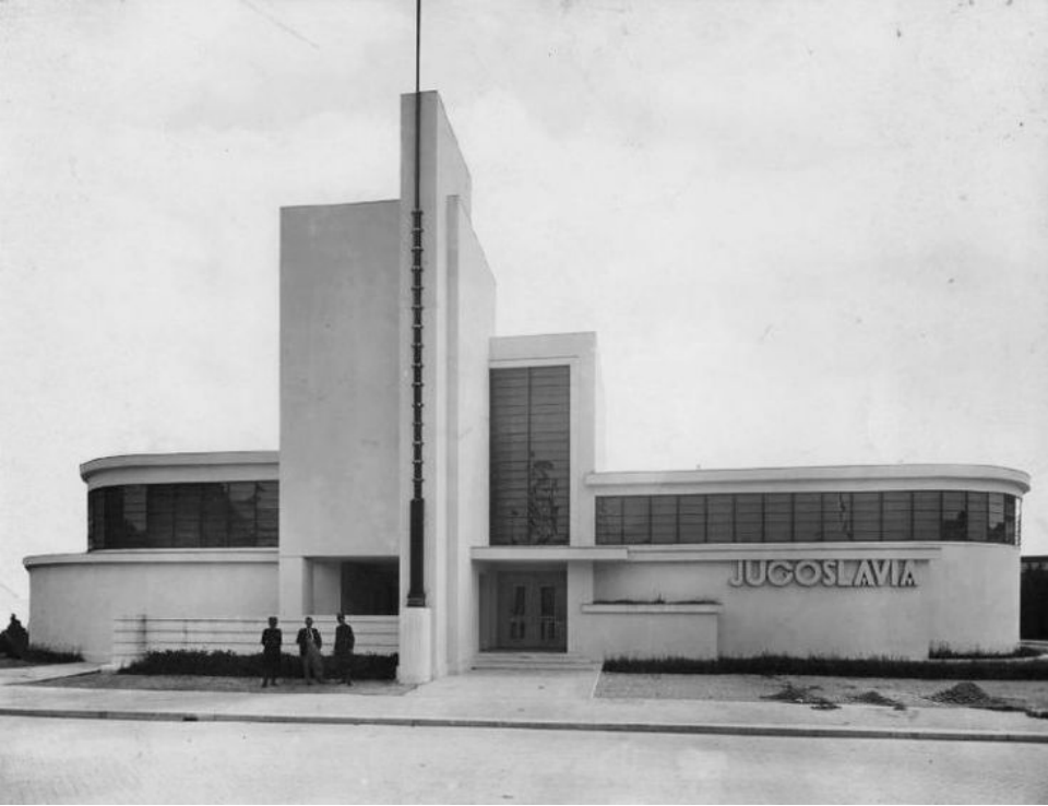
Драгиша Брашован, павиљон Југославије у Милану, 1931.
