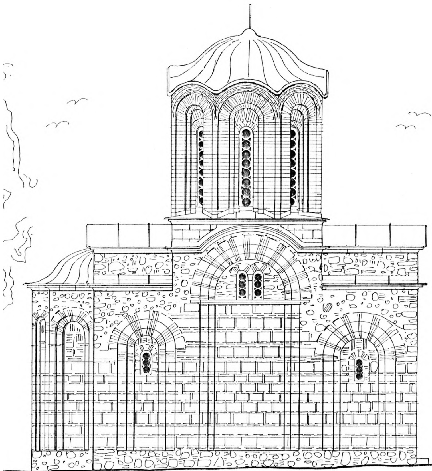
Црква Светог Никите, изглед са севера (цртеж: арх. Никола Ничота)
