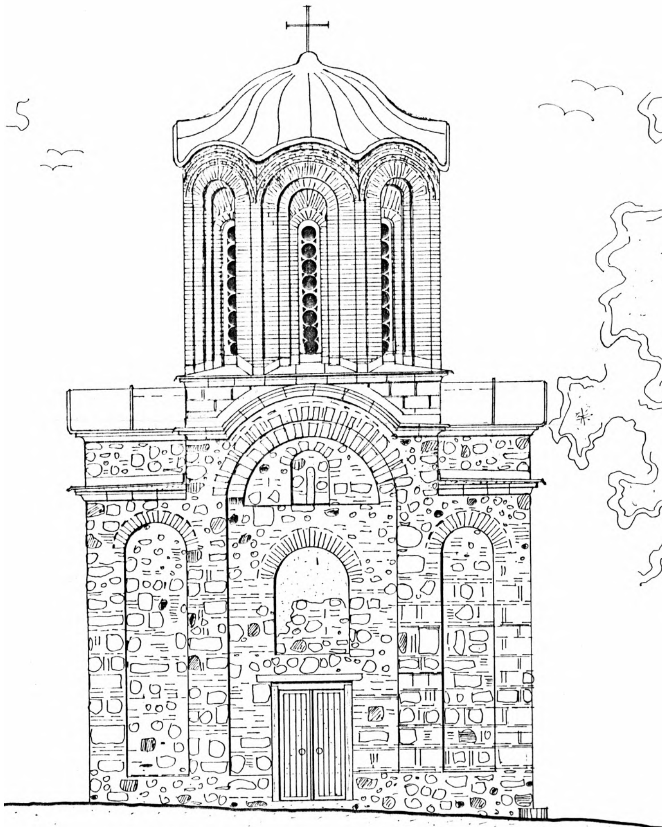
Црква Светог Никите, изглед са запада (цртеж: арх. Никола Ничота)
