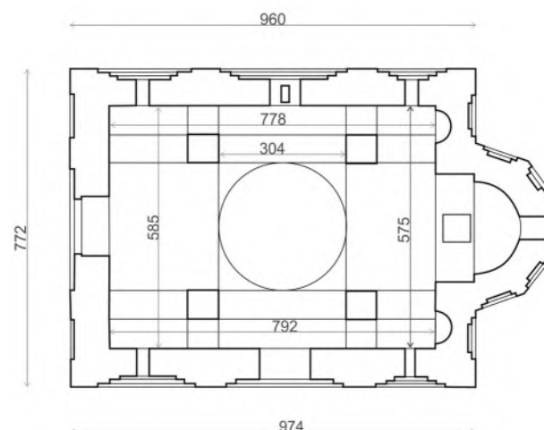
План цркве Светог Никите с котама (цртеж: Г. Толић)
