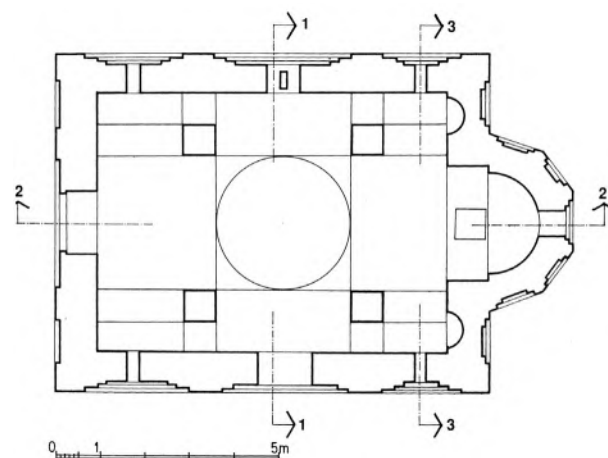
План цркве Светог Никите (према: Кораћ, Сјоменици)
