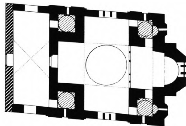
Основа цркве Светог Пантелејмона у Нерезима код Скопља, 1164. (према: S. Ćurčić, Architecture in the Balkans from Diocletian to Süleyman the Magnificent , New Haven 2010)
