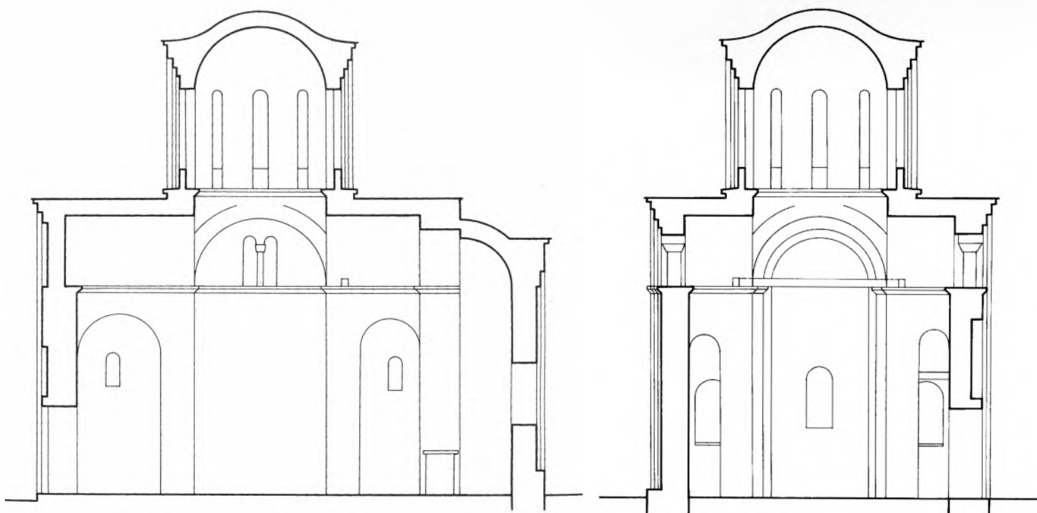
Подужни пресек цркве Светог Никите (према: Кораћ, Сѿоменици ) (лево); попречни пресек цркве Светог Никите (према: Кораћ, Сѿоменици ) (десно)
