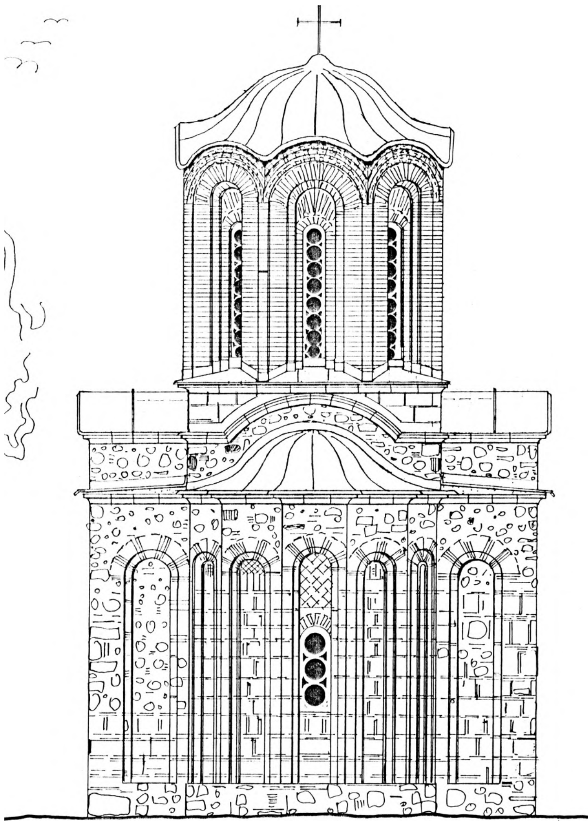
Црква Светог Никите, изглед са истока (цртеж: арх. Никола Ничота)
