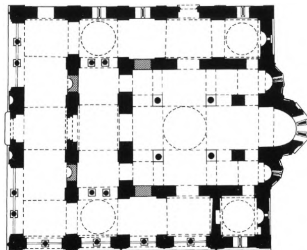
Основа цркве Светих апостола у Солуну, око 1315. (према: Ćurčić, Architecture in the Balkans )
